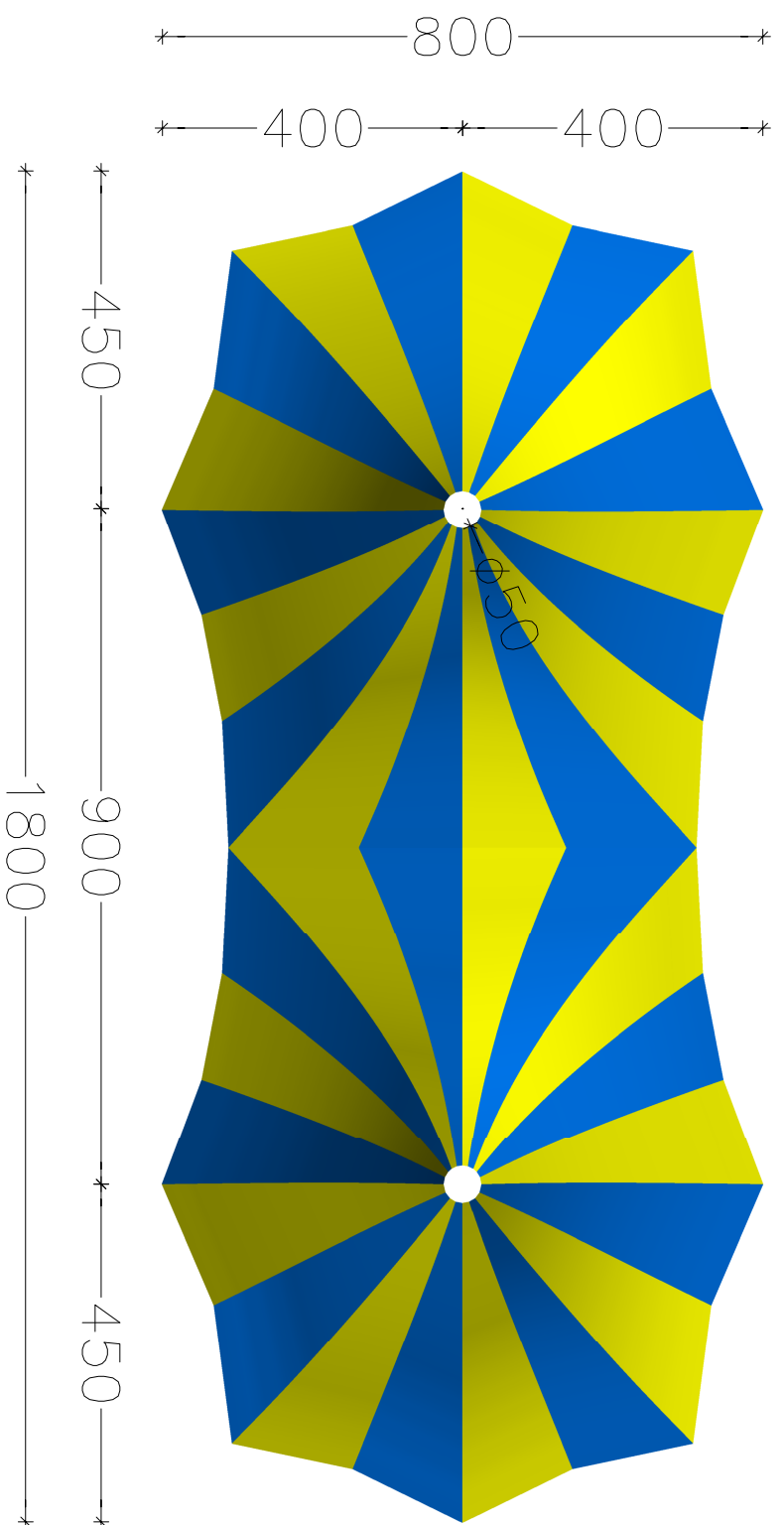
Pianta
