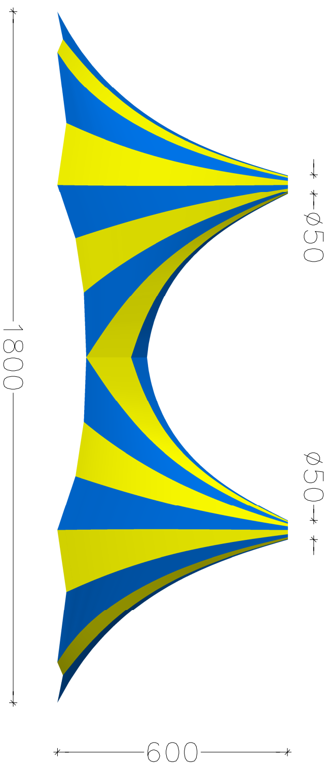
Vista frontale
